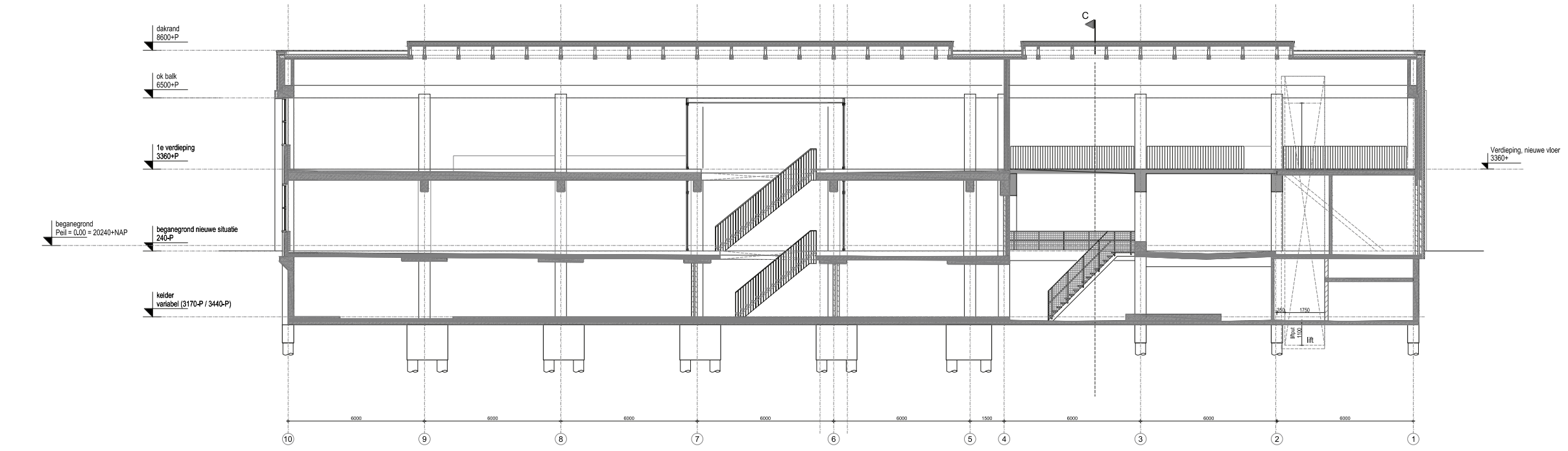
Doorsnede A-A
