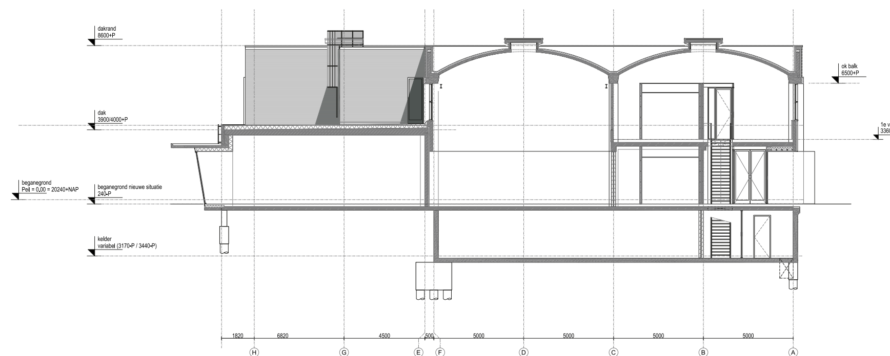
Doorsnede D-D
